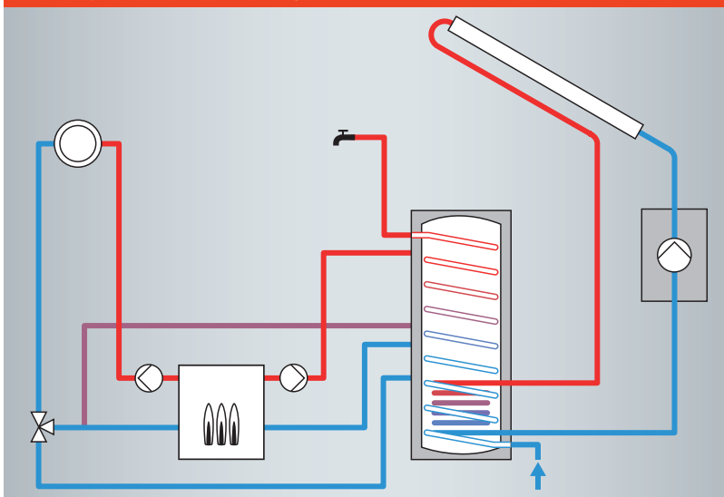
Abb. 6 System mit Rücklaufanhebung
