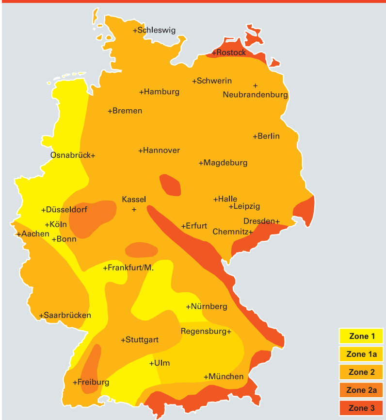
Abb. 1 Schneelasten
