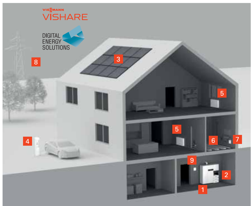
Regeneratives Energiesystem mit Brennstoffzellen-Heizgerät Vitovalor PT2, Stromspeicher-System Vitocharge sowie Photovoltaik-Anlage Vitovolt für eine hohe Unabhängigkeit vom öffentlichen Stromversorger.
