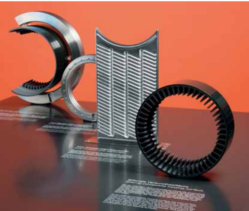
Innovationen im Bereich Wärmetauscher: von der biferralen Verbundheizfläche bis zum Inox-Radial-Wärmetauscher
